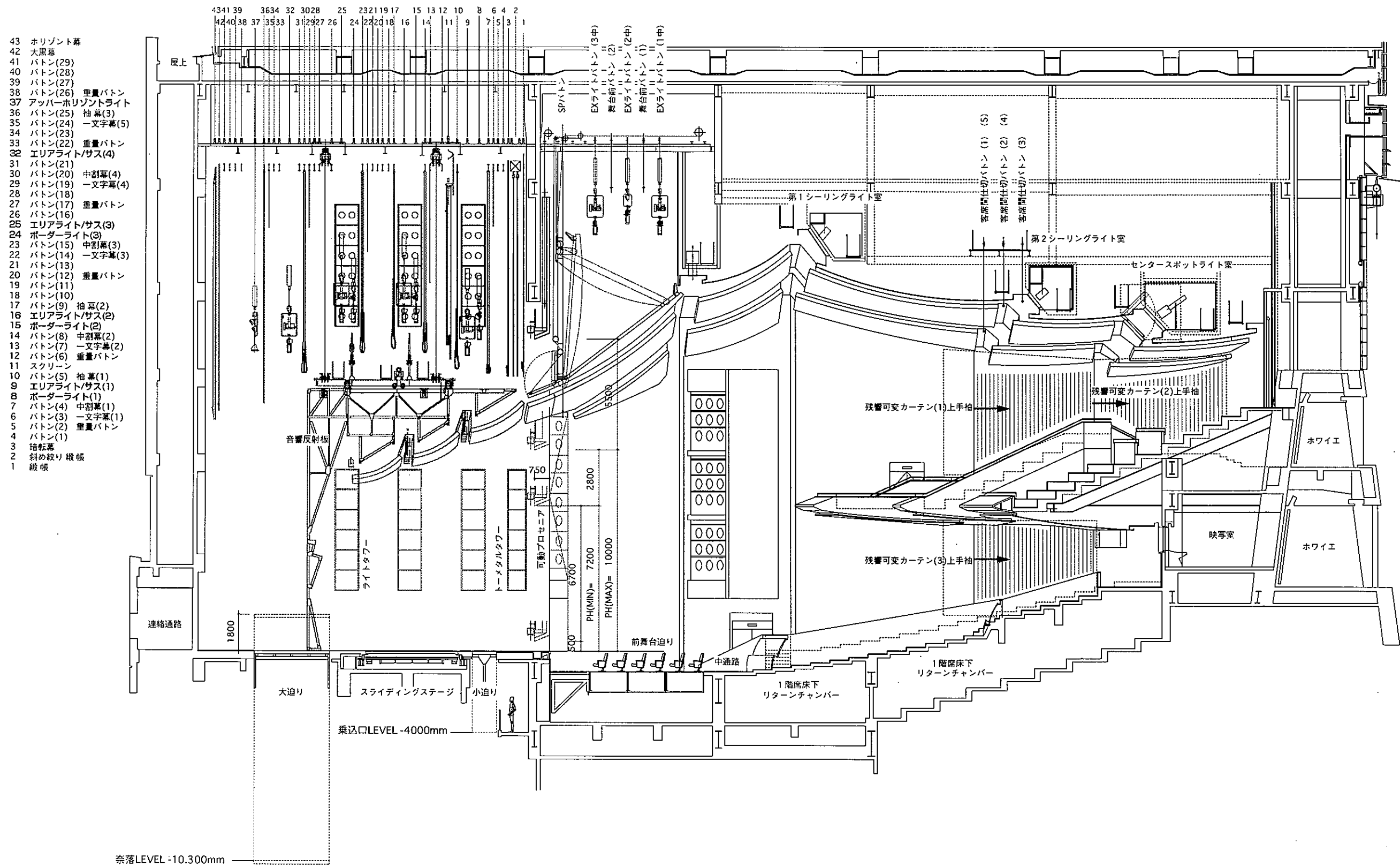
NHK 大阪ホール会場断面図(SCALE 1/200)
